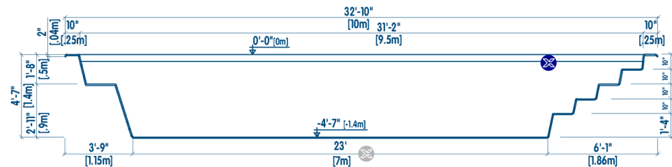
CORTE LONGITUDINAL | LONGITUDINAL SECTION
